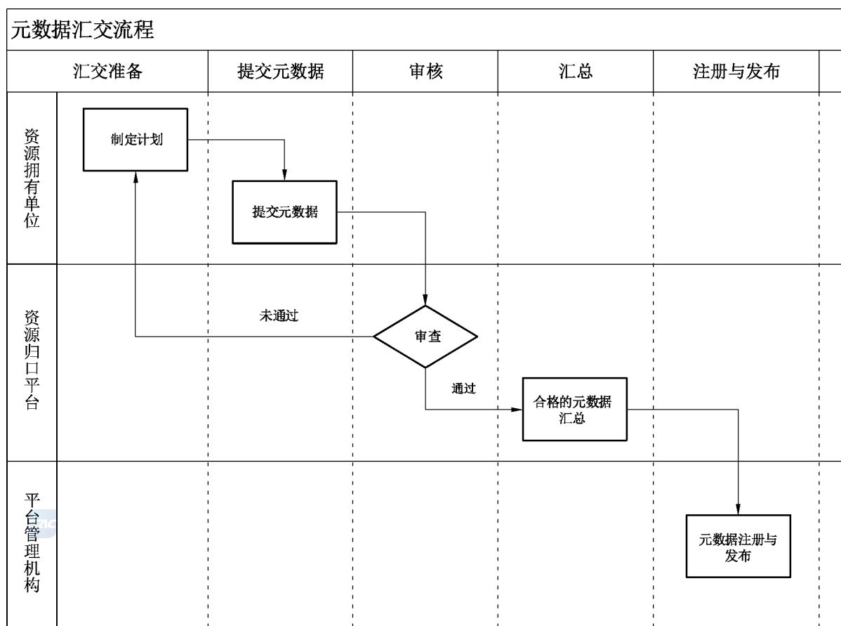
图 1 元数据汇交流程
